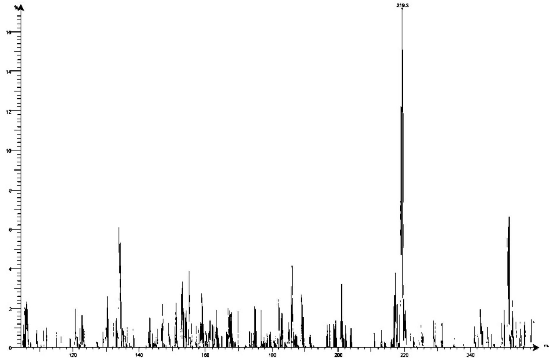
附 2：质谱
