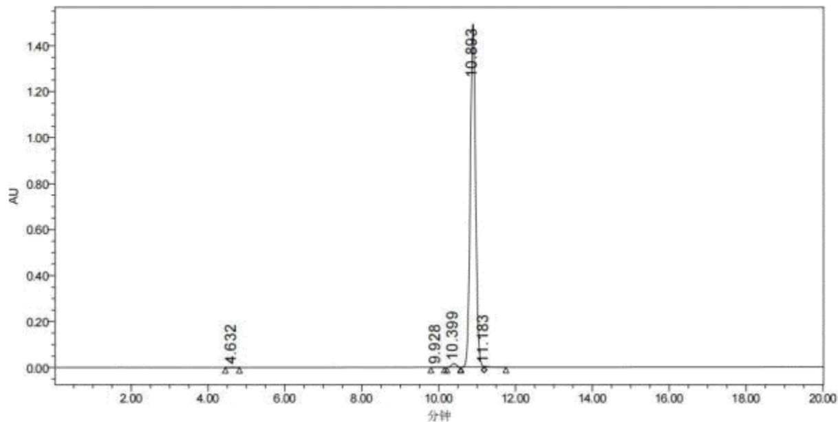
色谱峰结果
